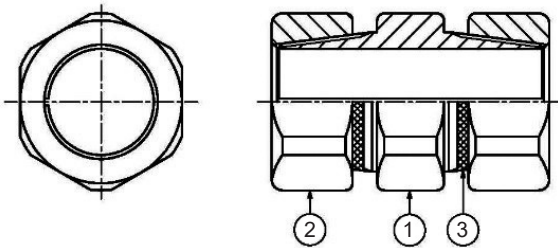
(図-1) 1. ボディ 2. ナット 3. シールテープ
